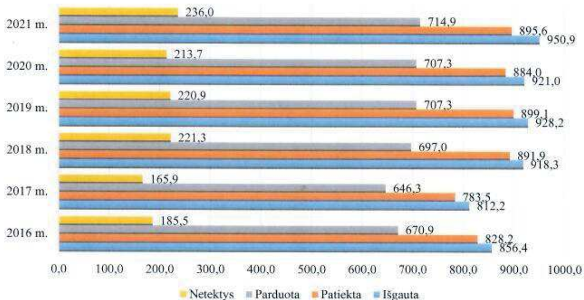
2 pav. Vandens tiekimas, realizacija, netektys, tūkst. m 3
